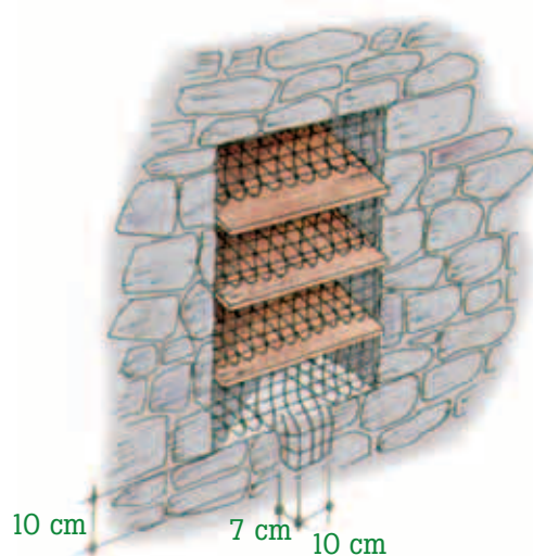
Schéma d'une nasse pour permettre la sortie des pigeons après obturation des abat-sons
