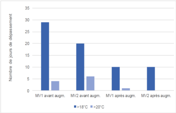
Figure 21 : Nombre de jours de dépassement des seuils de 18 et 20°C avant et après augmentation du débit réservé sur les deux stations du moyen Verdon (température maximale journalière)
