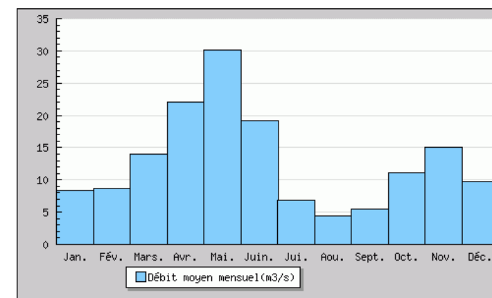
Verdon à Demandolx – 1948-2015
