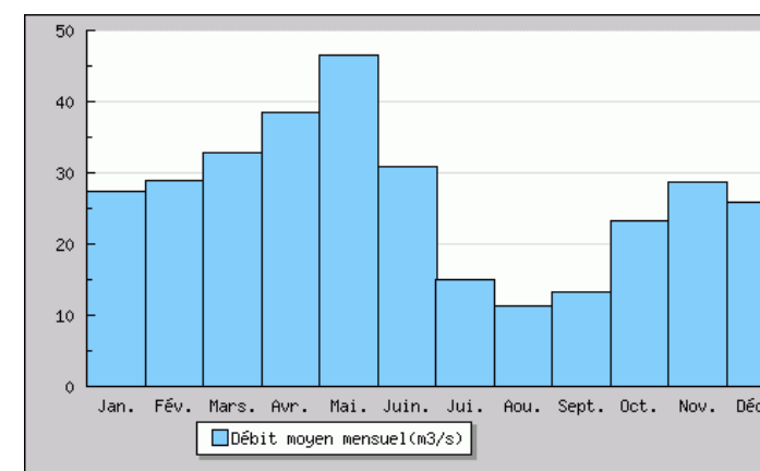
Verdon à Vinon – 1969-2015
