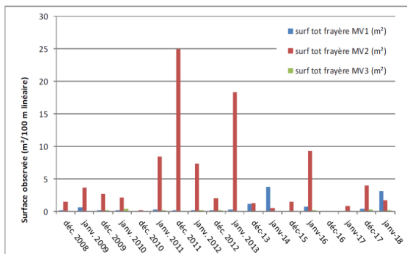
Figure 42 : Evolution des surfaces observées de frayère / 100 m linéaire de cours d'eau (période 2009 – 2018) sur les trois stations du moyen Verdon
