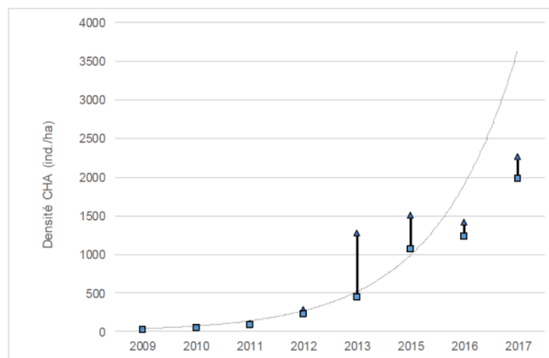
Figure 53 : Evolution des densités de chabots sur la station MV2 entre 2009 et 2017
