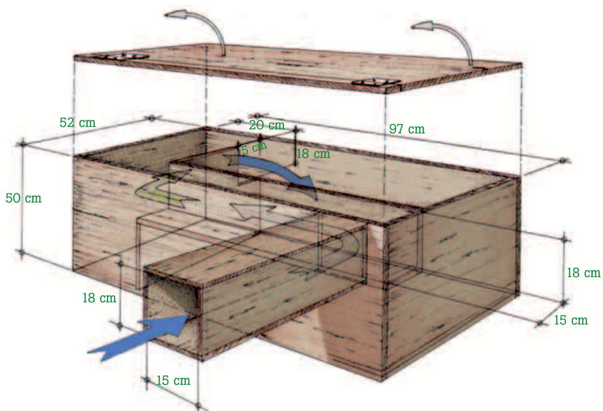
Schéma d'un nichoir avec galerie d'accès à chicane intérieure (d'après J. De Boe)
