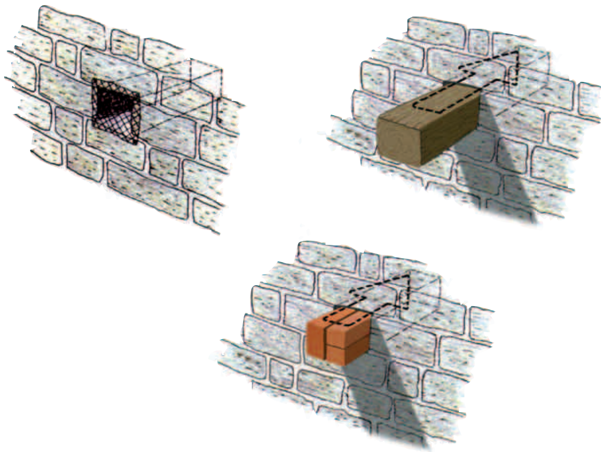
Schémas d'obturation des trous de boulin
