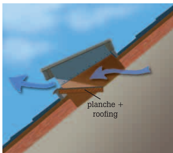
Avec planche d'envol
