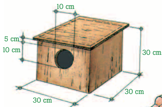
Schéma d'un nichoir
