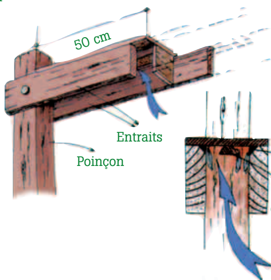
Construction entre entrails parallèles
