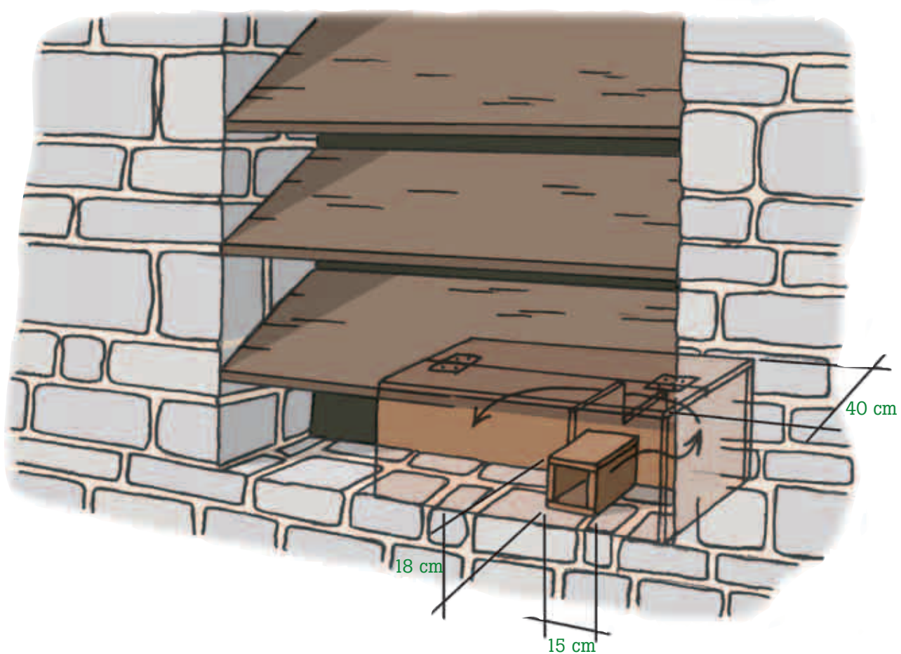
Schéma d'un nichoir avec galerie d'accès simple
