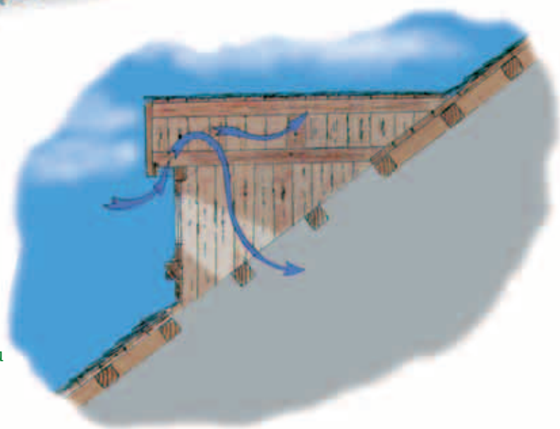
Ouverture pratiquée sur le fronton
