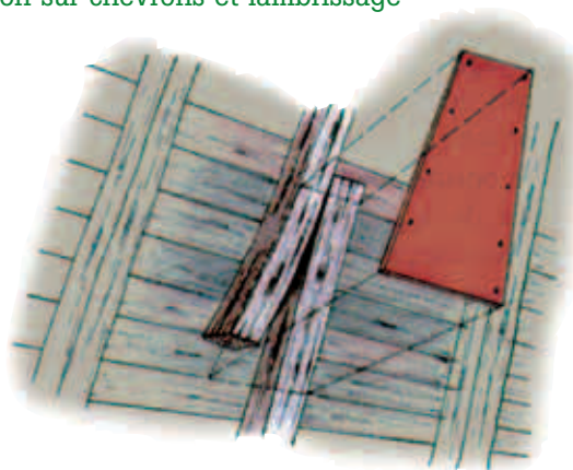
Construction sur chevrons et lambrissage
