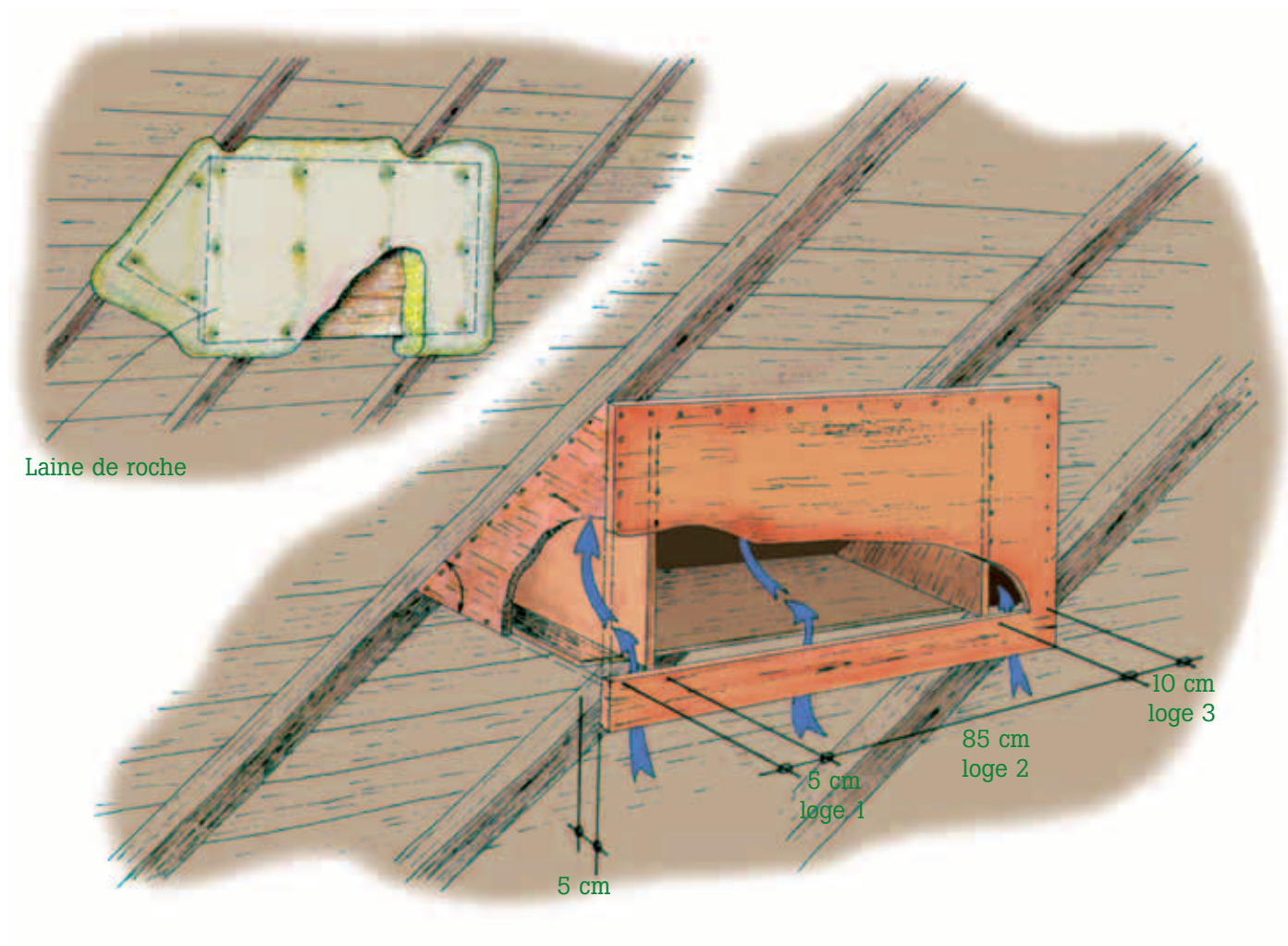
Schémas de construction
