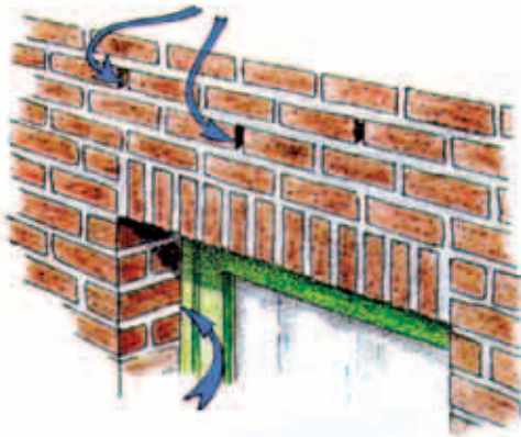
Accès par un joint resté ouvert dans le mur de parement
