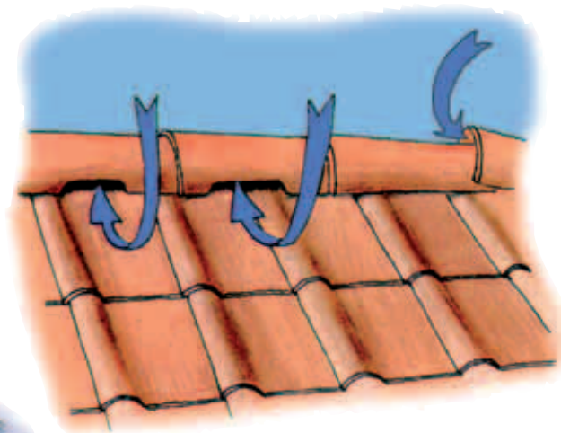
Fentes à la base de tuiles faîtières
