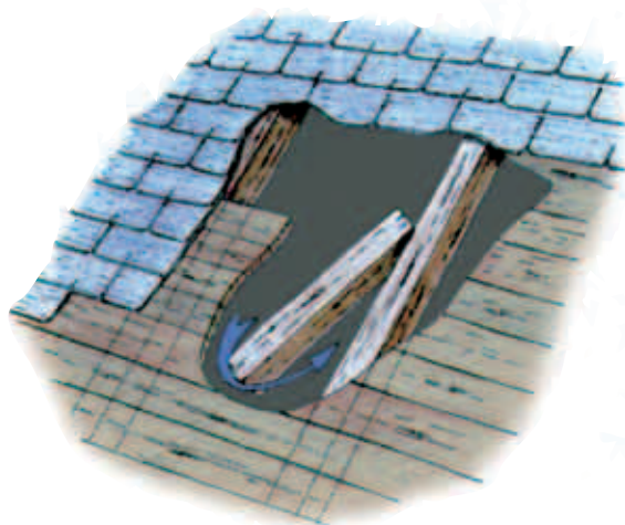
Construction sur chevrons et lambrissage
